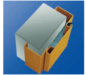
Variofix Stahlzarge Verzinkt, grundiert (pulverbeschichtet)
